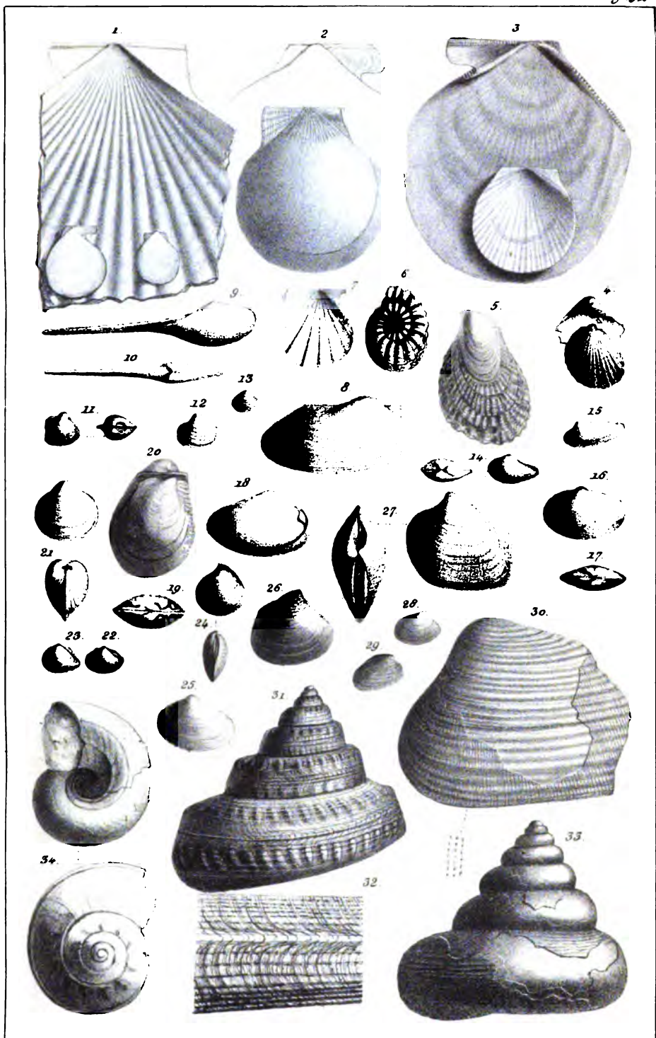
Queenstede, Jura.
